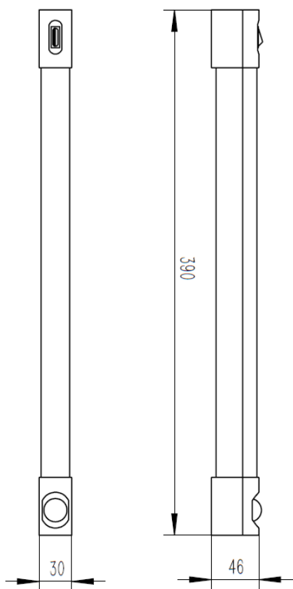
外形尺寸图纸
